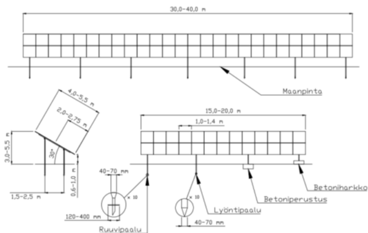
KUVA. Telineen tyypipiirustus ja perustusesimerkkejä
