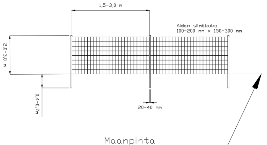
KUVA. Tyypikuva aidasta
