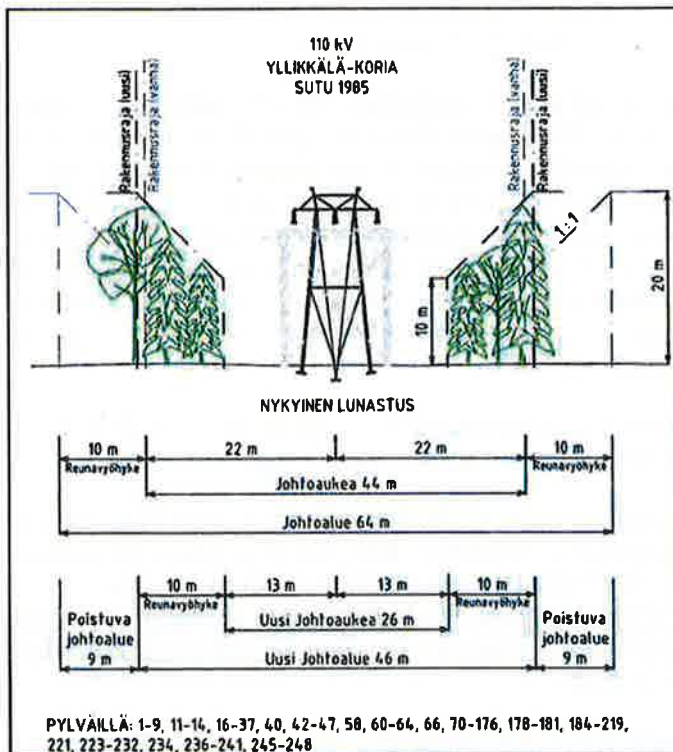
Kuva 1. 110 kV voimajohdon poikkileikkaus tulevassa tilanteessa.
